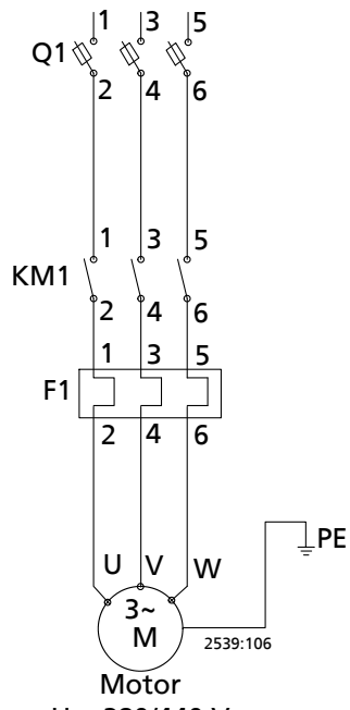
Abb. 19: Drehstromausführung
