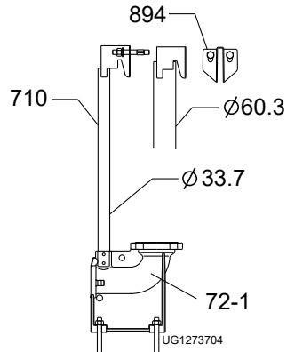
Afb. 8: 1 geleidebuis monteren
