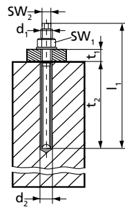
Fig. 5: Dimensões
