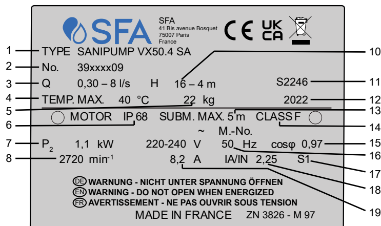
Afb. 2: Typeplaatje (voorbeeld)
