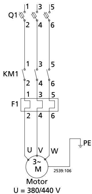
Fig. 19: Versione a corrente trifase
