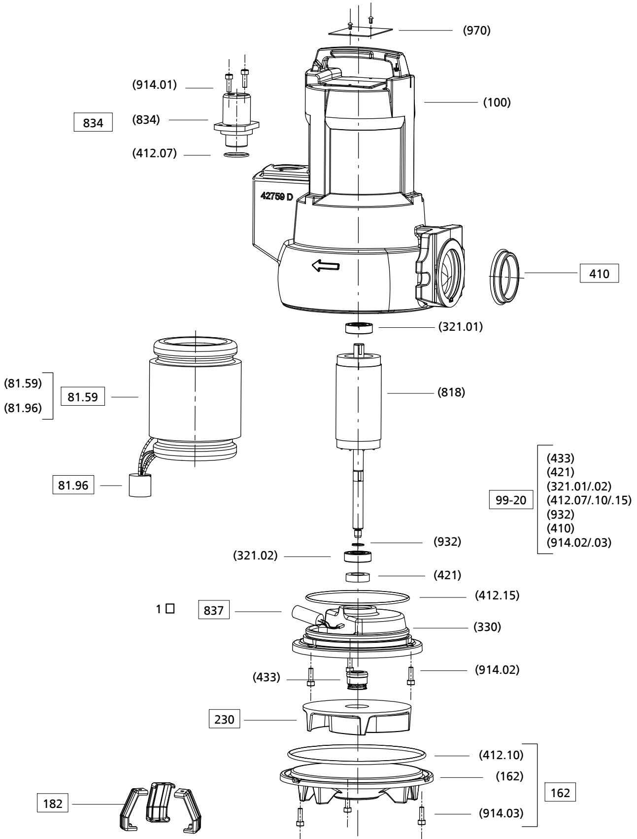
Fig. 16: Disegno esploso Sanipump VX
