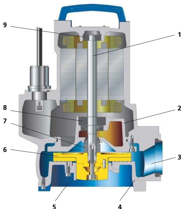
Fig. 3: Disegno di sezione
