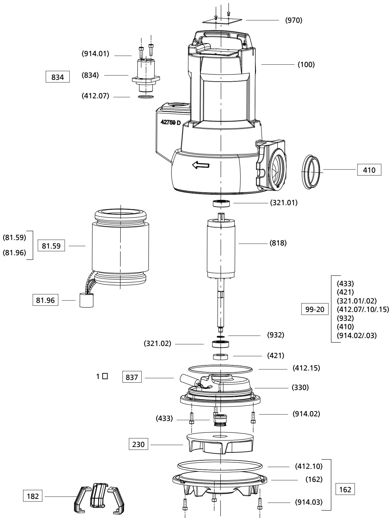
III. 16: Vue éclatée Sanipump VX
