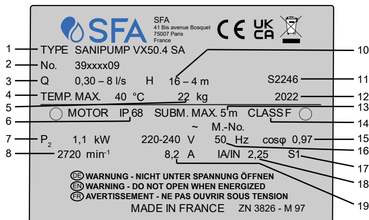
Fig. 2: Placa de características (exemplo)
